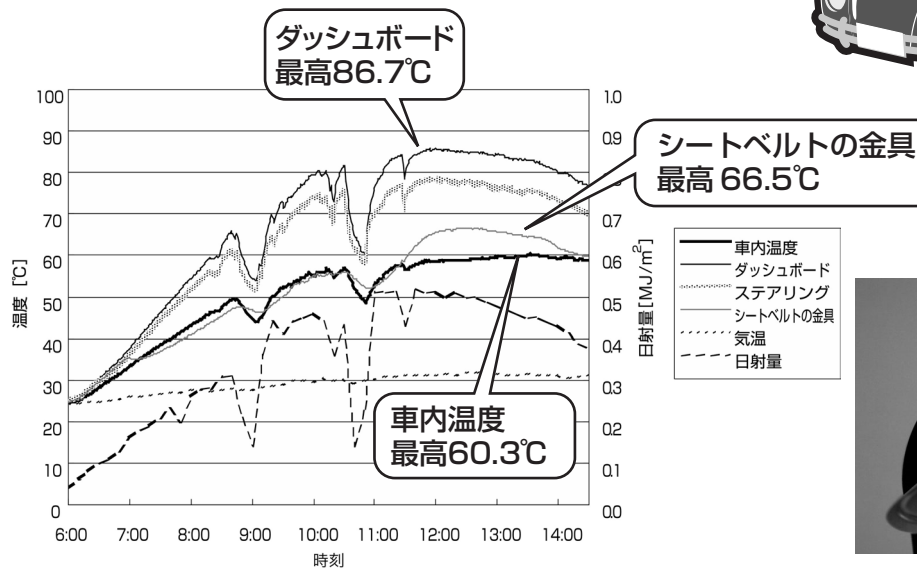
図1 車内各部の温度上昇例 (ウィンドウ全閉の場合)
